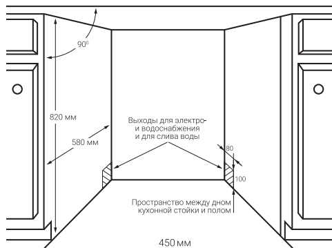
Рис. 1 Размеры кухонной стойки менее 5 мм между верхней частью машины и кухонной стойкой. Дверца должна быть вровень с кухонной стойкой
