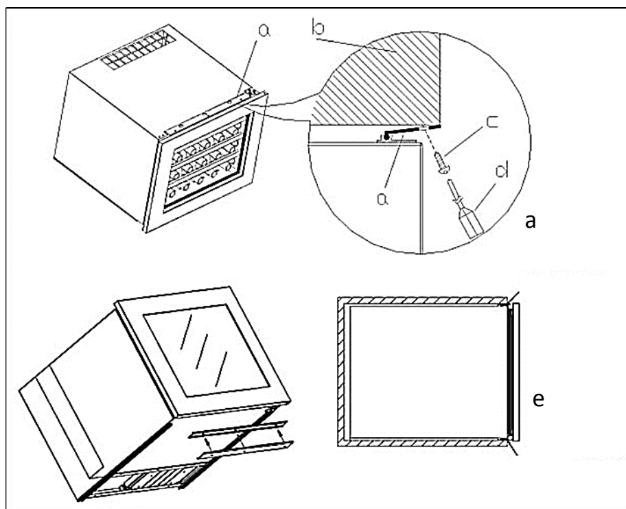
а. Верхний фиксатор б. Винный шкаф с. Винт d. Отвертка e. Нижний фиксатор
