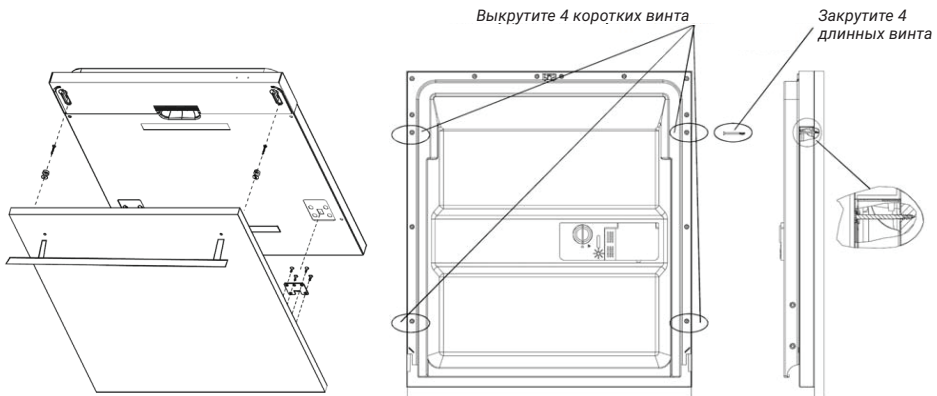
Рис. 4 Установка внешней панели
